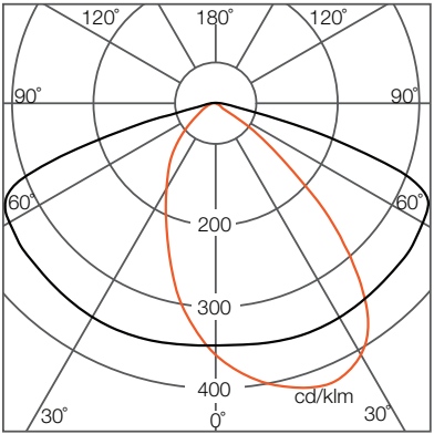
SMB ( 路灯配光 Type II )
